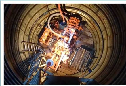
全油圧駆動 二重管式穿孔機K1-B
